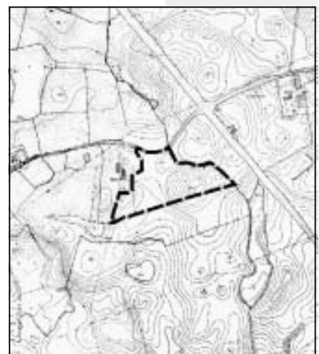
Skizze: Geltungsbereich des B-Plans Nr.5 der Gemeinde Wahlstorf
